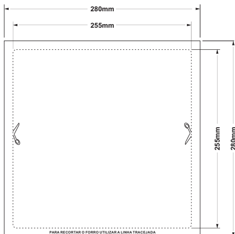
Dimensões para recorte do forro
